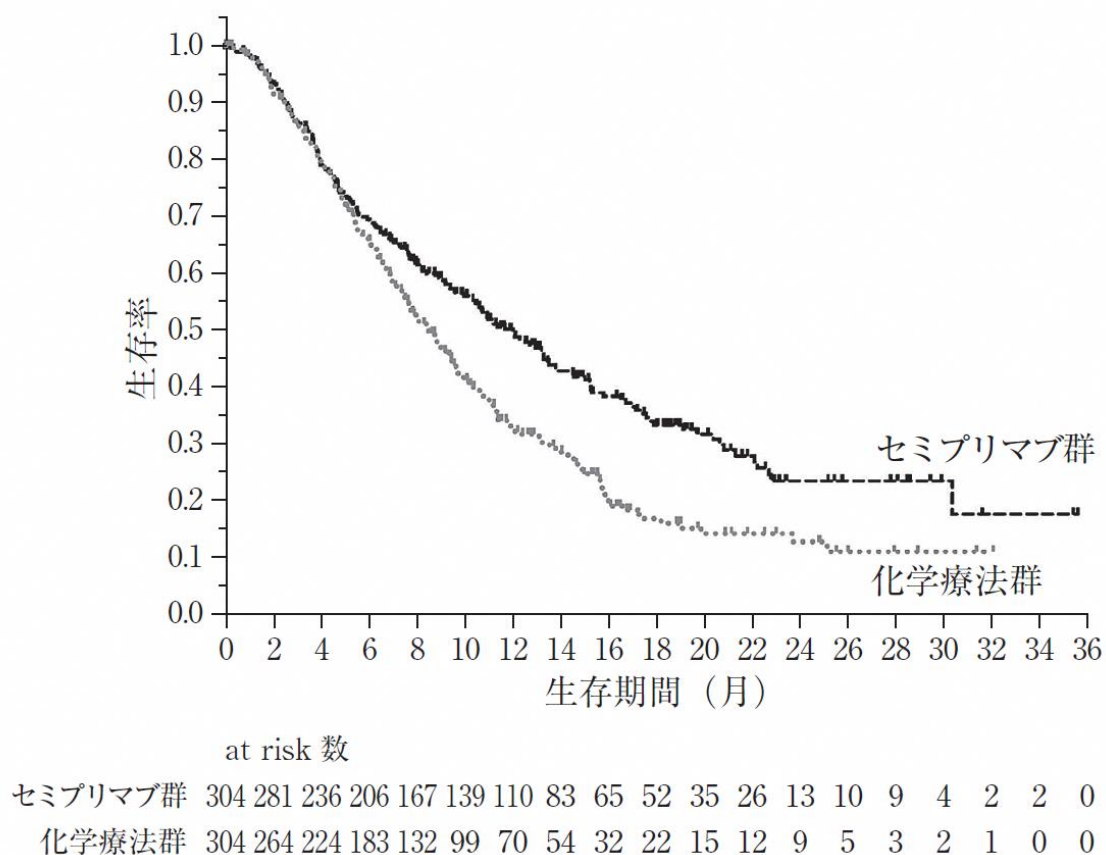
図1 OSのKaplan-Meier曲線 (R2810-ONC-1676試験)
